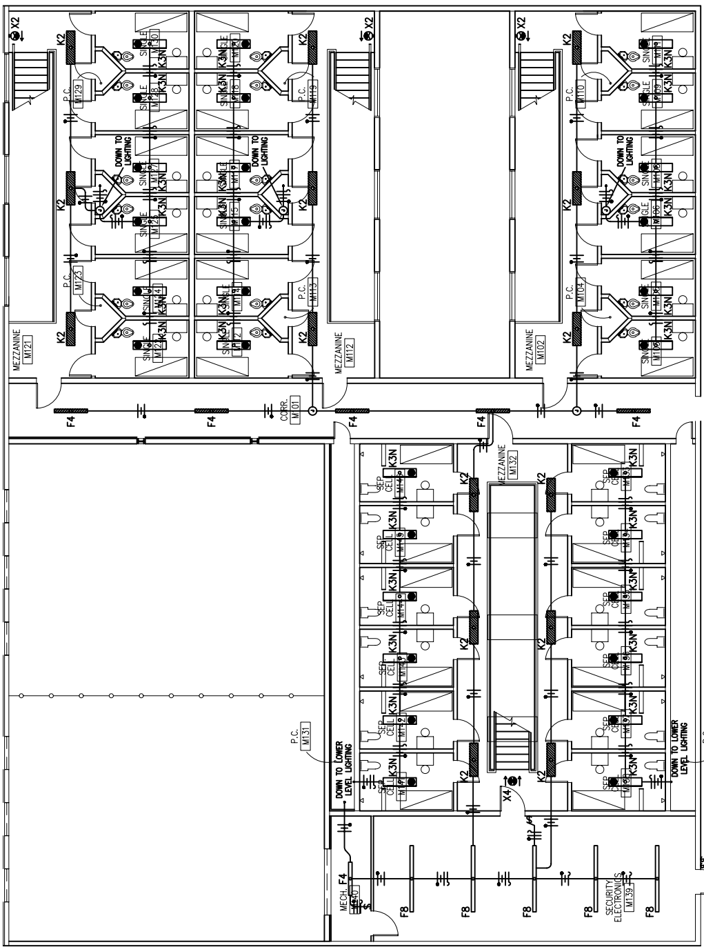
MEZZANIN SCALE: 1/16" = 1'-0" E2.00 2
